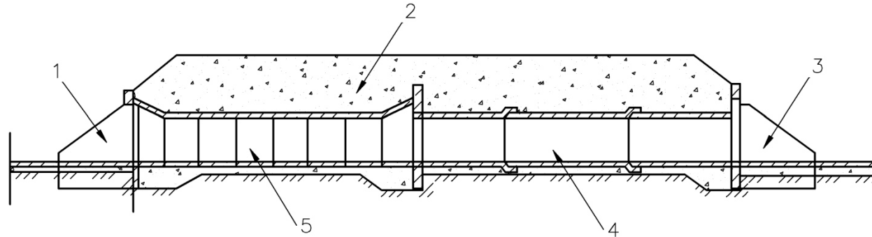
Рисунок 5.3.1. Общий вид водопропускной трубы:
